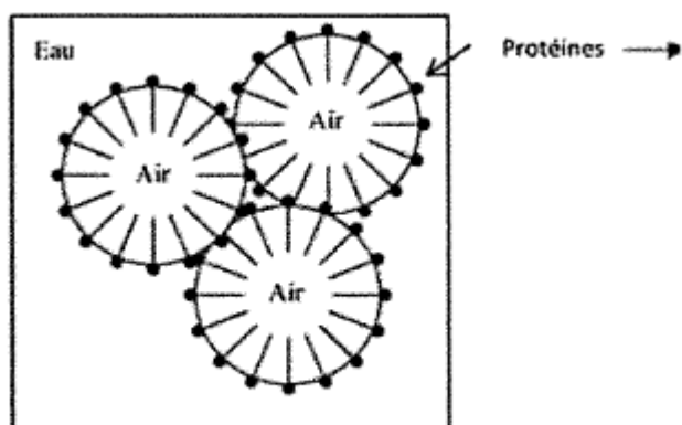
Organisation des protéines dans une mousse air-eau
